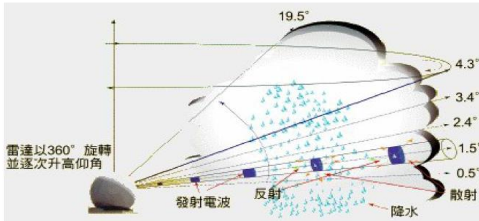
图4-2 雷达探测示意图
