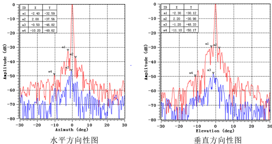
图4-4 天线方向性图
