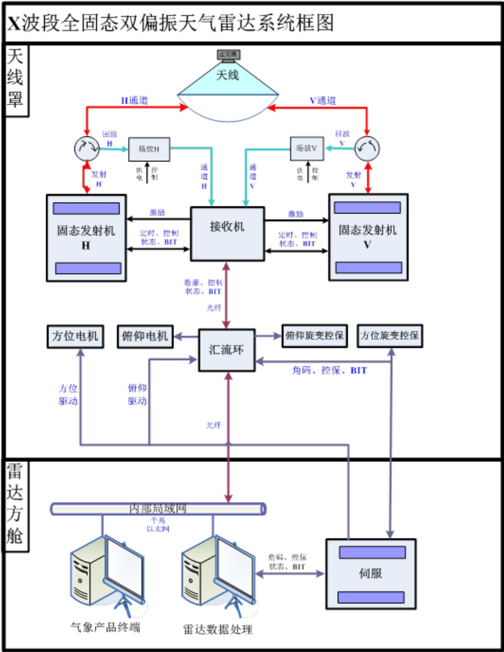
图4-5 系统工艺流程图
