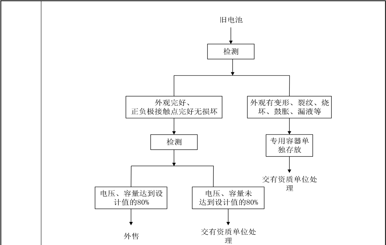
图 2-4 再生新能源动力蓄电池生产工艺流程
