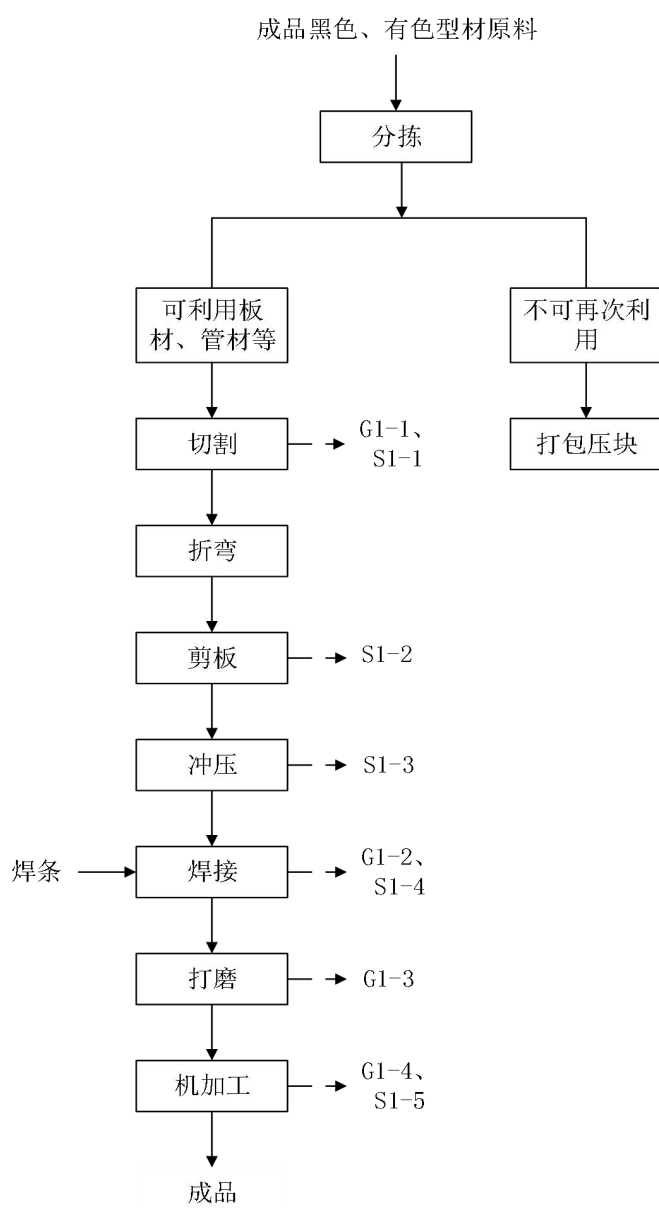
图 2-2 再生金属冲压件制品生产工艺流程
