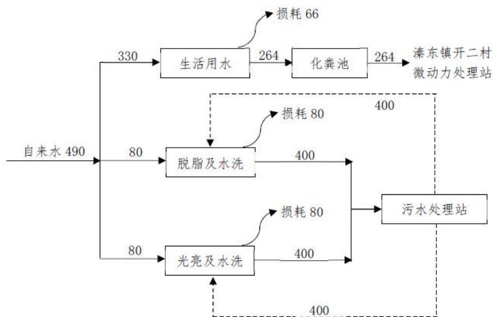
图 2-1 扩建项目水平衡图（单位：吨/年）
