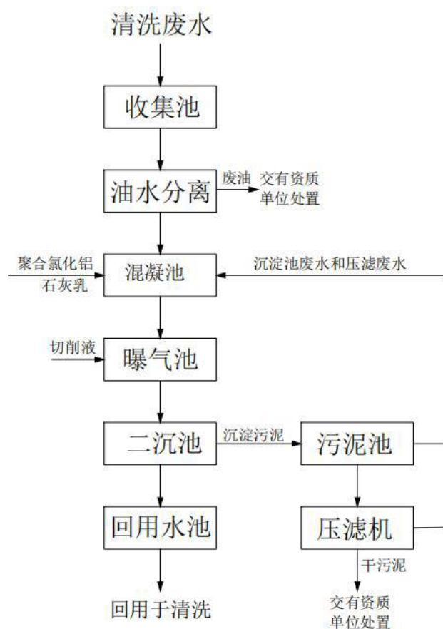
图 4-4 东台市华威标准件有限公司工业废水处理流程图
