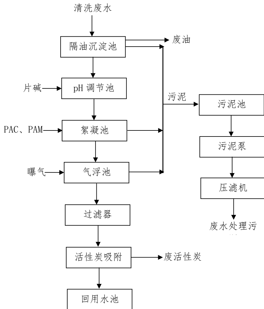
图 4-3 清洗废水处理工艺流程图
