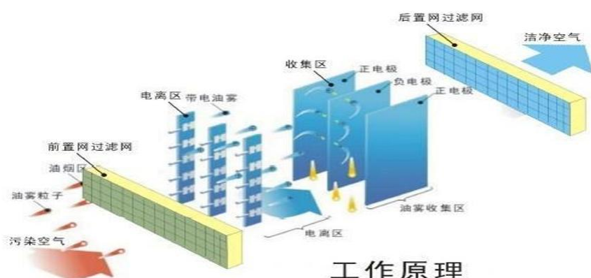
图 4-2 静电式油烟净化器工作原理图
