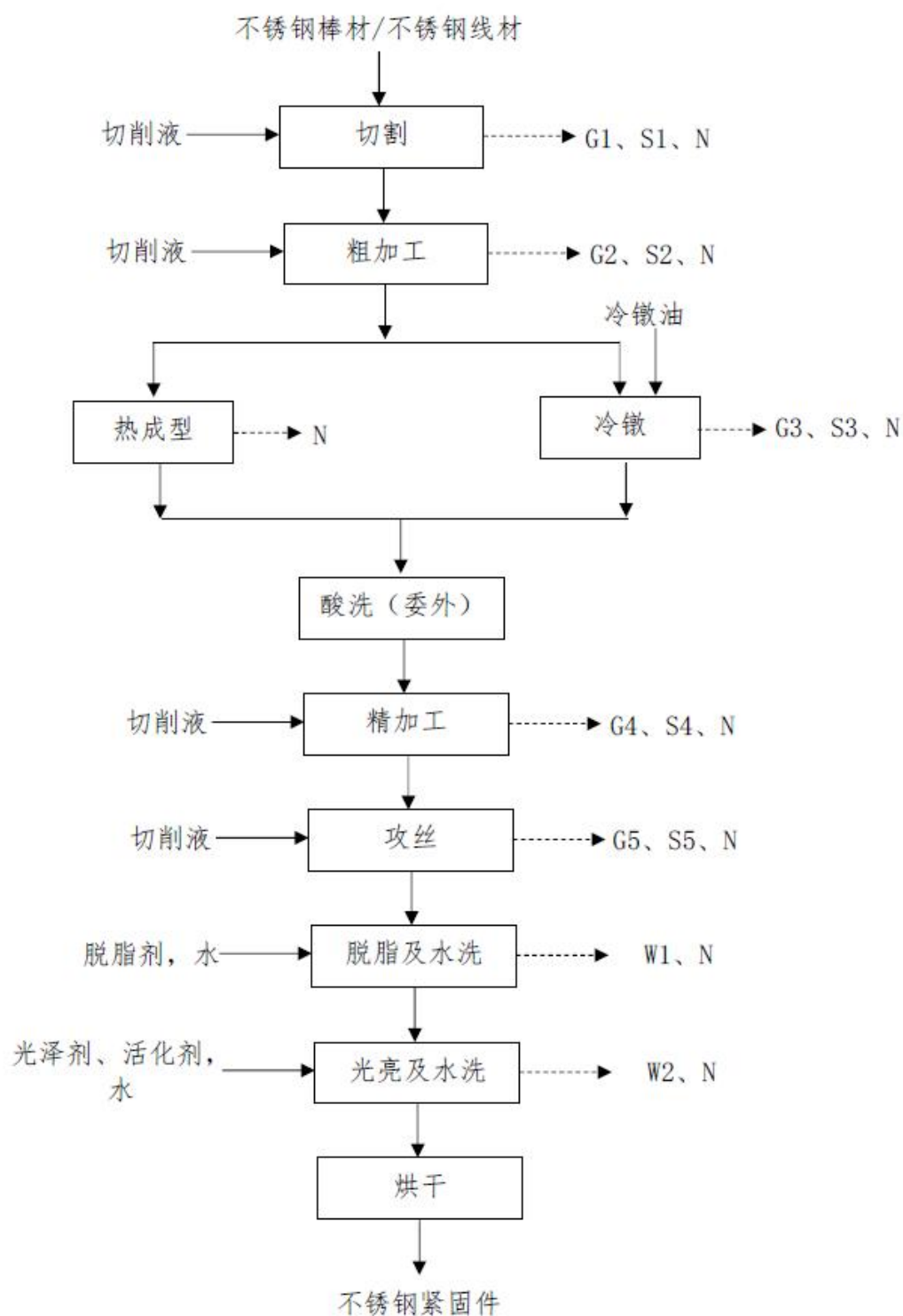
图 2-4 扩建项目生产工艺流程及产污节点图
