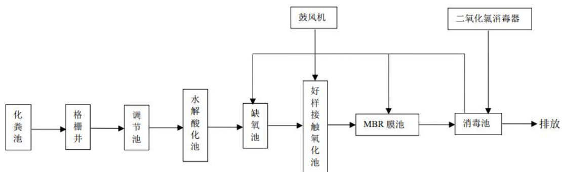
图 4-5 溱东镇开二村微动力处理站污水处理工艺流程
