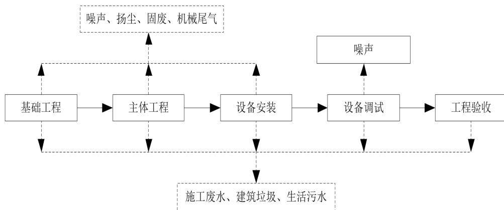
图 2-3 施工期工艺流程及产污情况图
