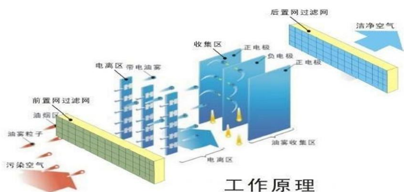
图4-2 静电式油雾分离器工作原理图
