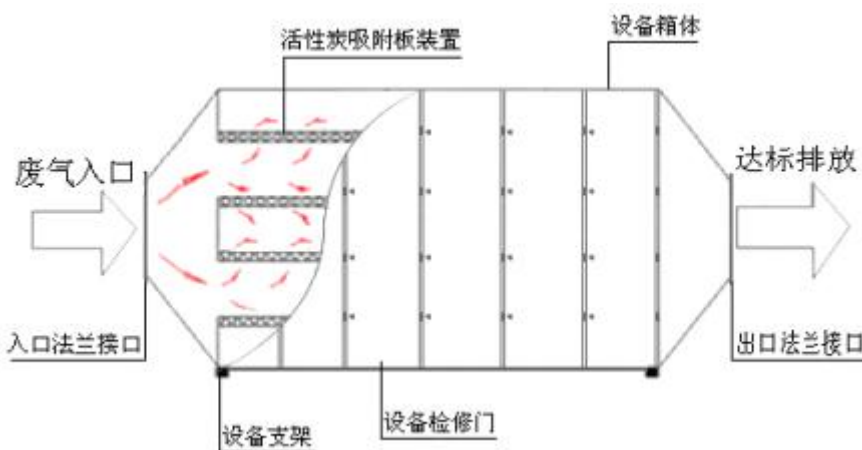
图4-3 活性炭吸附装置工作图
