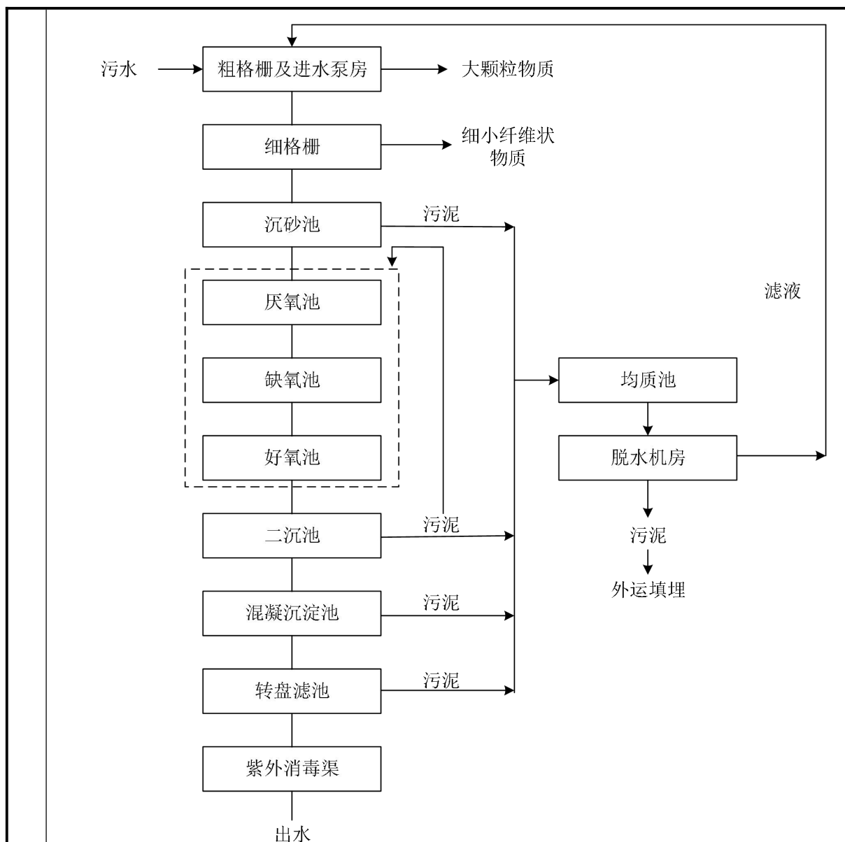
图 4-4 东台市溱南污水处理有限公司处理工艺流程图
