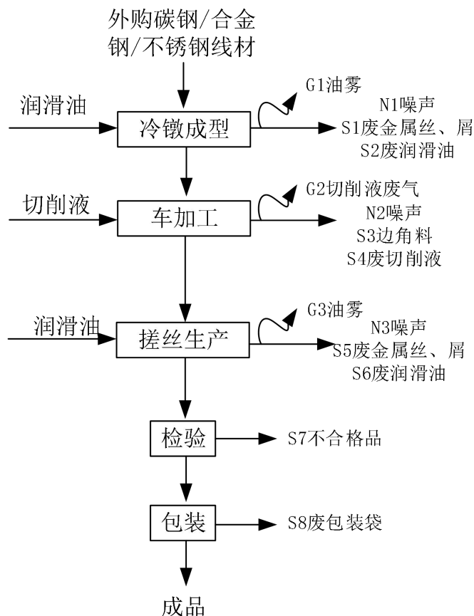
图 2-2 特种合金紧固件生产工艺流程图及产污环节图
