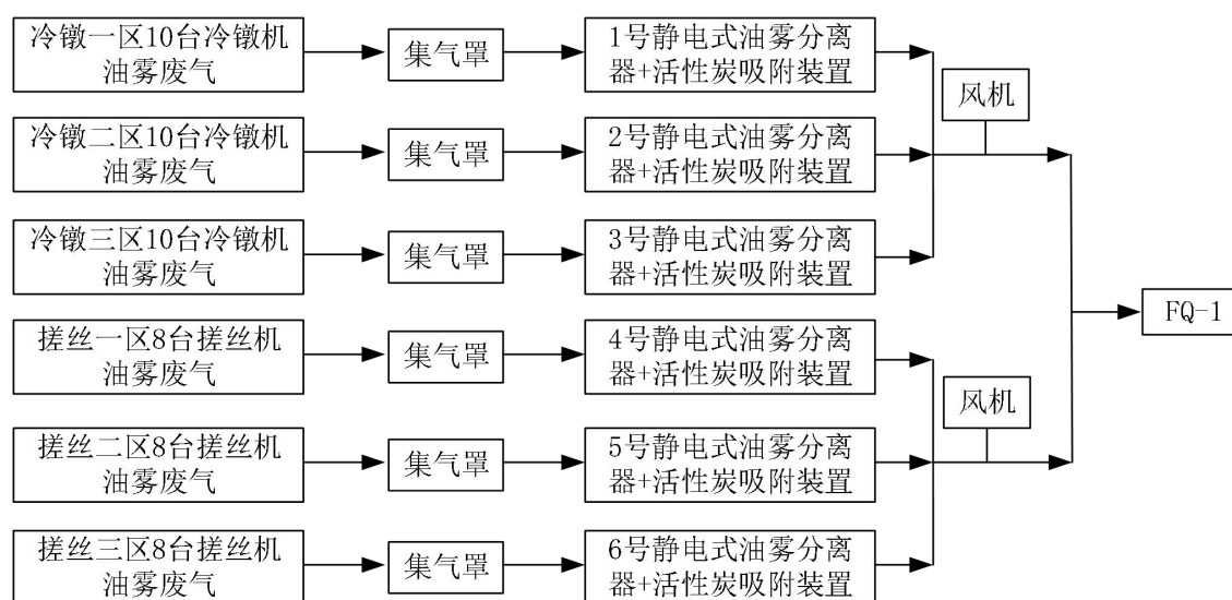
图4-1 本项目有组织废气处理工艺流程图
