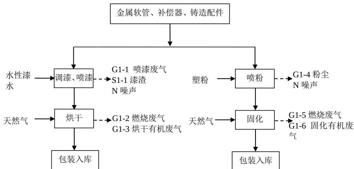
图 2-5 喷涂工艺及产污流程图
