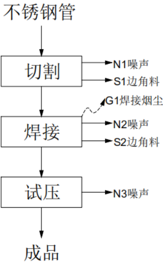
图 2-8 补偿器产品生产工艺流程及产污环节图
