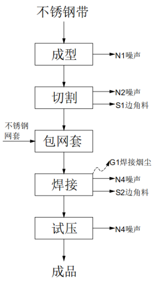
图 2-6 金属软管产品生产工艺流程及产污环节图
