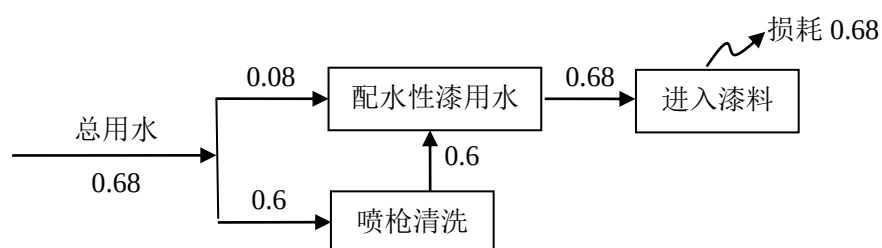
图 2-1 本项目给排水平衡图 (t/a)
