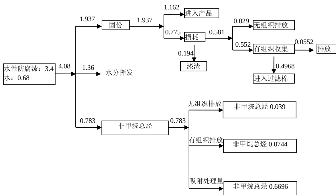
图 2-3 项目水性防腐漆物料平衡图 (单位: t/a)
