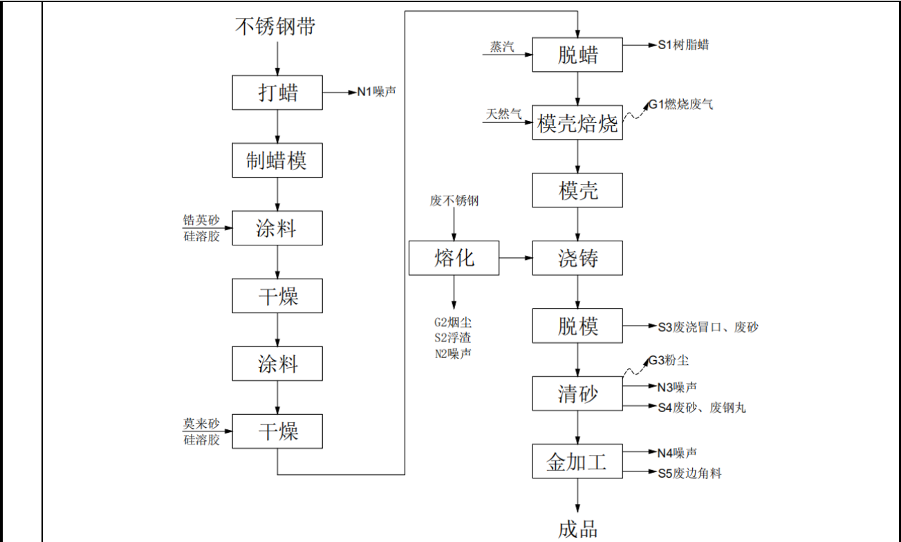
图 2-8 铸造配件产品生产工艺流程及产污环节图
