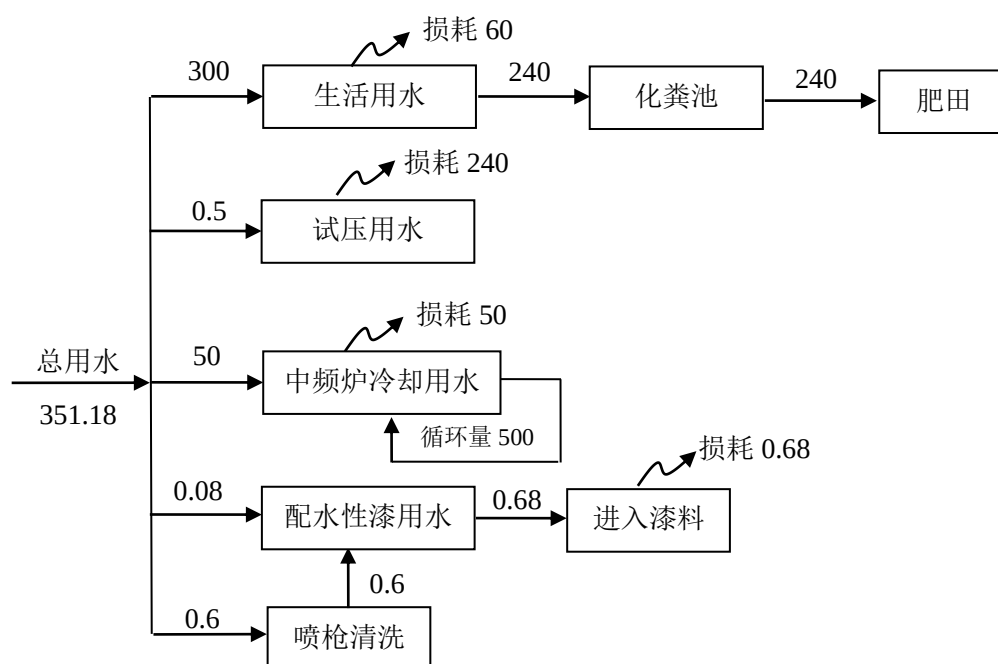
图 2-2 技改后全厂给排水平衡图 (t/a)
