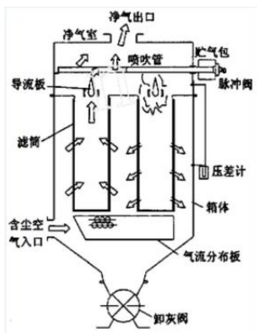
图 4-1 滤筒除尘装置工作原理图
