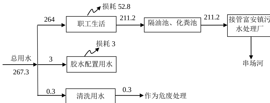
图 2-1 建设项目给排水平衡图 (t/a)
