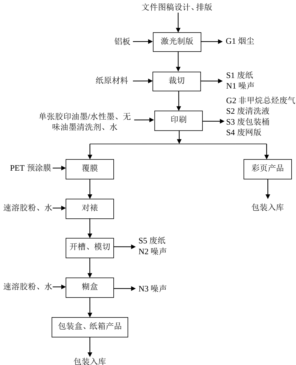
图 2-3 包装盒、纸箱、彩页生产工艺及产污流程图
