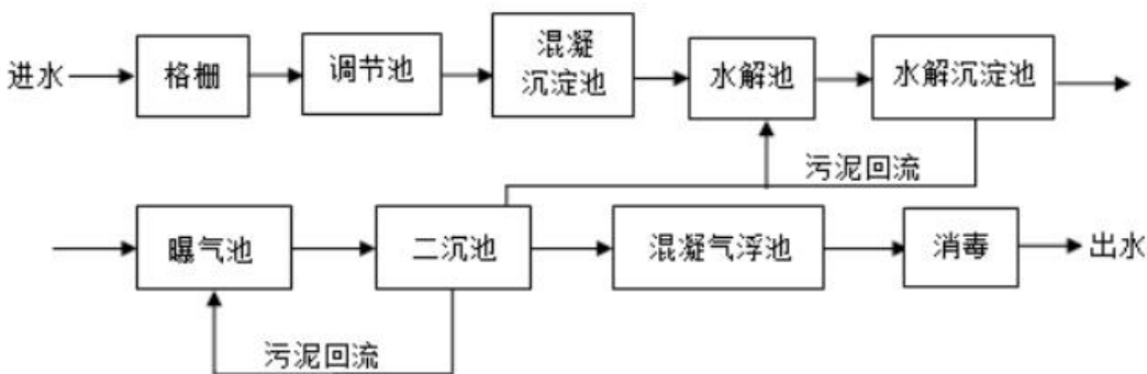
图 4.2-1 东台清源污水处理厂一期工程处理工艺流程图
