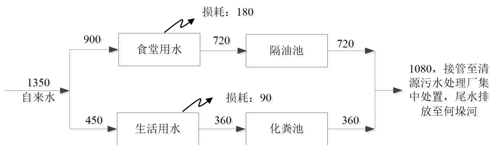
图 2.2-1 本项目水量平衡图（单位：t/a）
