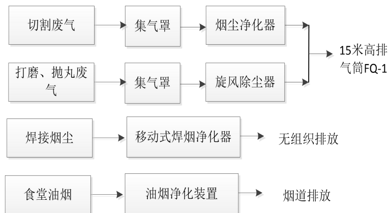
图 4.2-1 本项目废气处理工艺流程图
