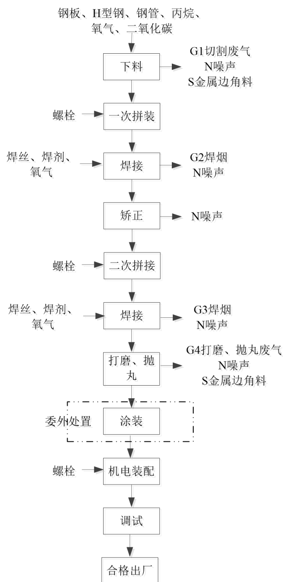
图 2.3-1 工艺流程图及产污环节图
